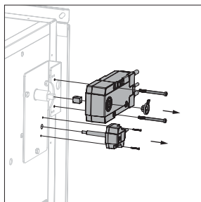
Type BFN(T) op CR2/CU2/ CU4/CU2-15:
