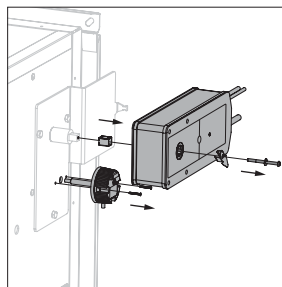
Type BFN(T) sur CR2/CU2/CU4/CU2-15:
